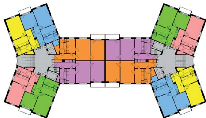
Půdorys typického podlaží
