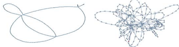
Obr. 3: Síť náhodného shluku znaků (vlevo) a úryvku rukopisu (350 slov)
