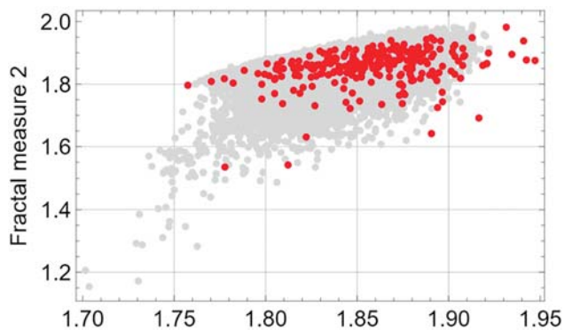
Obr. 4: Fraktální analýza rukopisu (červené tečky) a Hemingwayova románu Stařec a moře. Podle tohoto možná spadá rukopis do množiny přirozených jazyků. Zdroj: Ivan Zelinka
