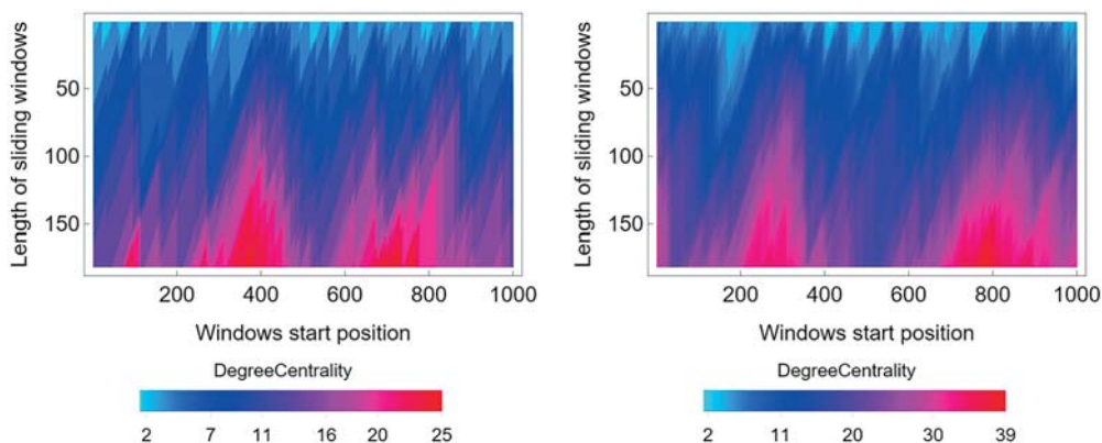
Obr. 2: Jiné zobrazení složitosti textu ve Voynichově rukopisu (vlevo) a v anglické verzi Bible (vpravo). Každý obrázek představuje 200 000 výpočtů.
